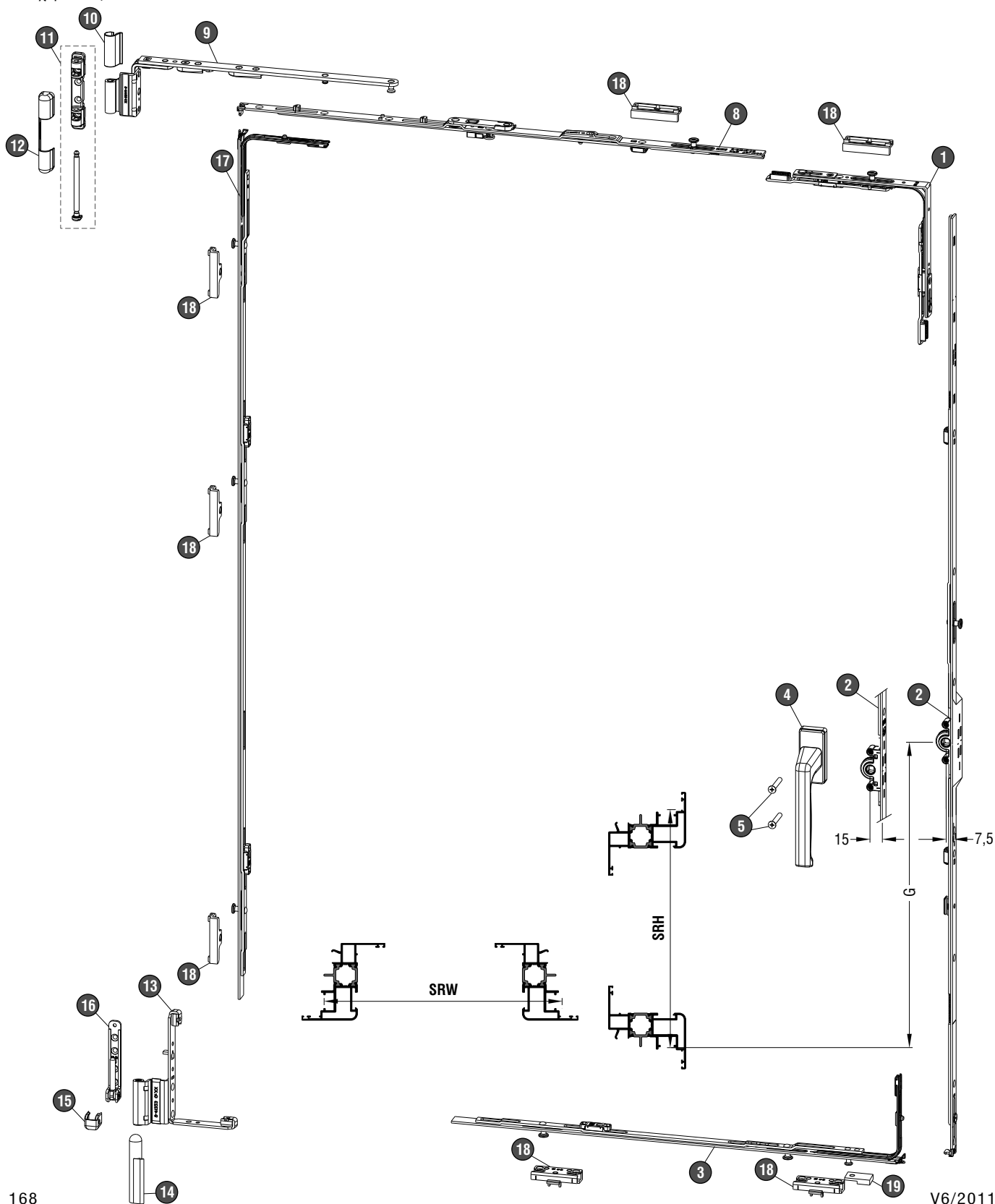
Δύο χερούλια | Two handles
