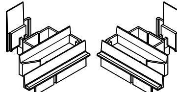
Τάπα μπινιού M20543 End cap for M20543 sash inversion profile
