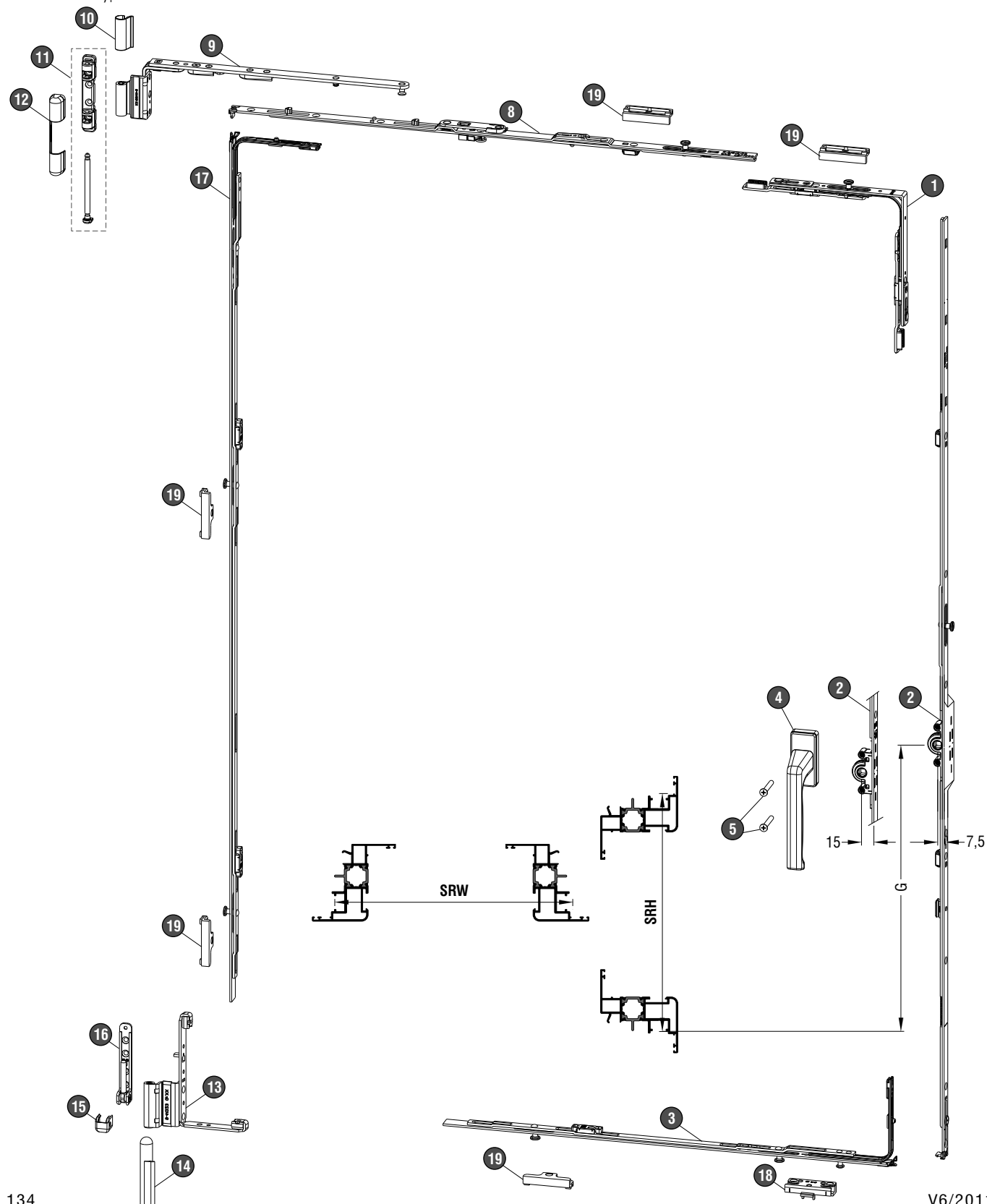
Δύο ανακλίσεις | Two tilt sashes
