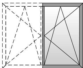
Δίφυλλο ανοιγόμενο - ανακλινόμενο (Πρώτο φύλλο) Two sash tilt & casement window (First sash)
