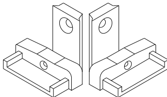
Τάπα κατωκασίου M15172 End cap for M15172 threshold profile
