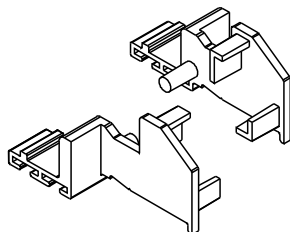
Τάπα πρόσθετου M20511 End cap for M20511 beauty profile
